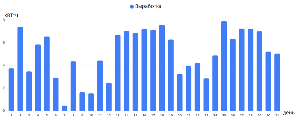
Рисунок 3.5 – Выработанная СФУ электроэнергия в мае 2021 по дням.
