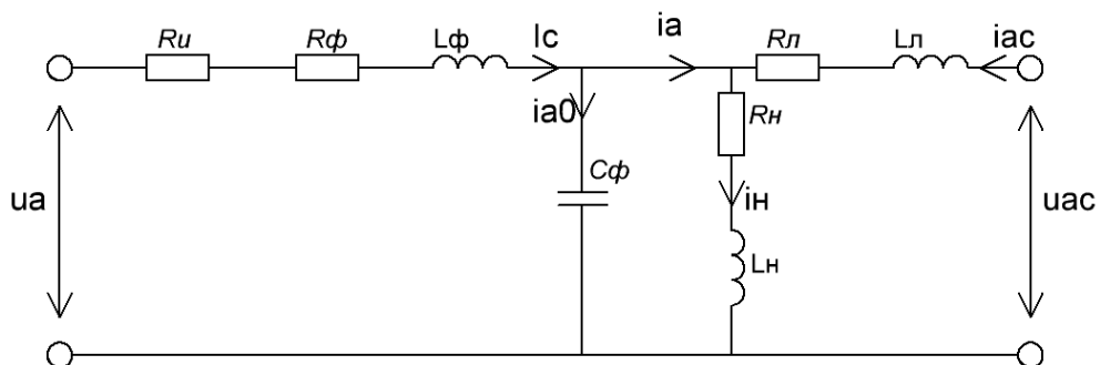
Рисунок 2.3 – Схема замещения фазы А
