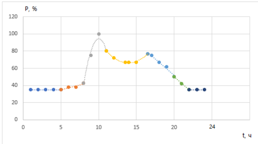
Рисунок 3.7 – Расчетный суточный график нагрузки потребителя
