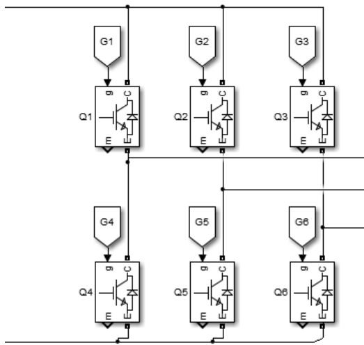
Рисунок 2.8 – Схема блока инвертора
