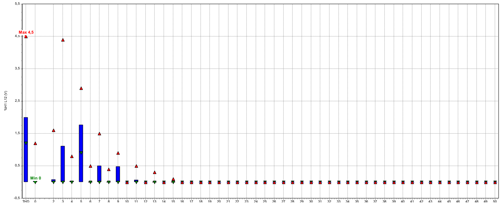
Гармонические искажения напряжения при отключенной солнечной электростанции
