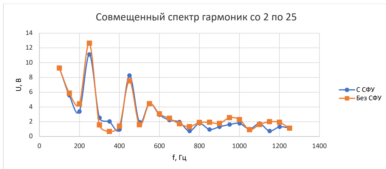
Рисунок 4.1 – Спектральный анализ напряжения у потребителя электроэнергии
