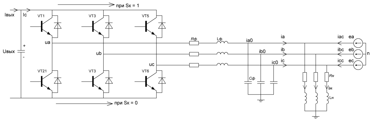
Рисунок 2.2 – Схема трехфазного сетевого инвертора
