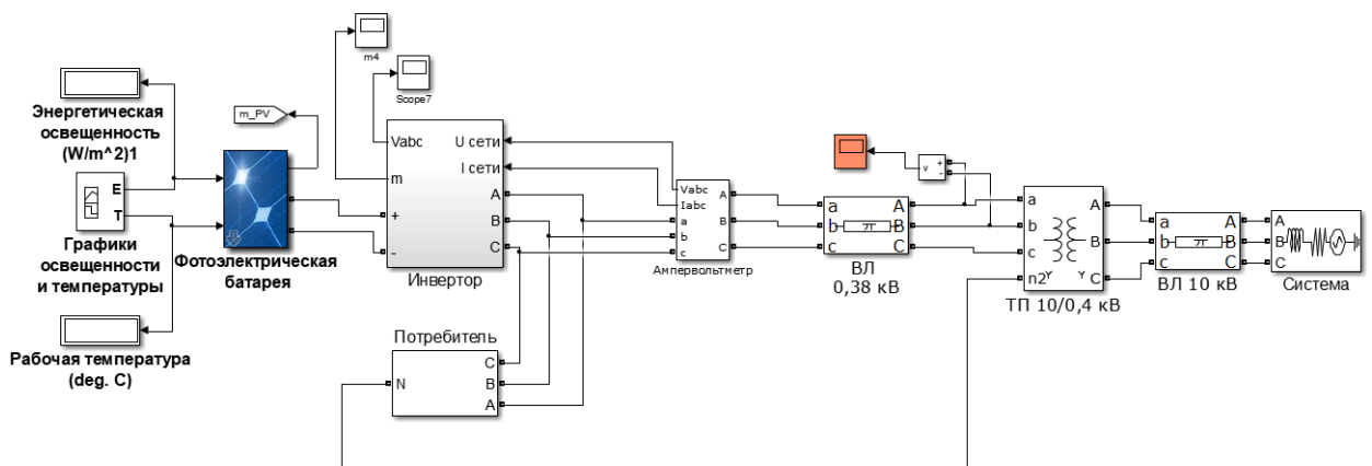
Рисунок 2.4 – Структурная схема имитационной модели СФУ, работающей параллельно с электрораспределительной сетью, для электроснабжения сельскохозяйственных потребителей
