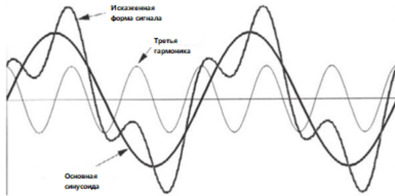
Рисунок 1.10. – Влияние 3-й гармоники
