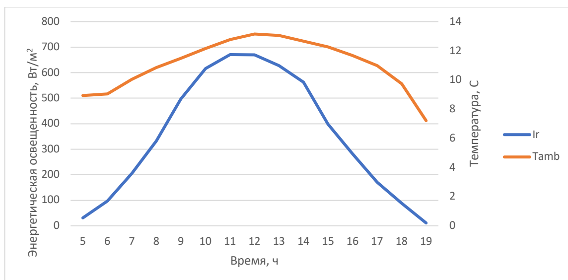
Рисунок 3.1 – Изменение энергетической освещенности и температуры окружающей среды 4 мая 2021 г., Саратовская область, р.п. Романовка, 51.750065 с.ш, 42.758712 в.д
