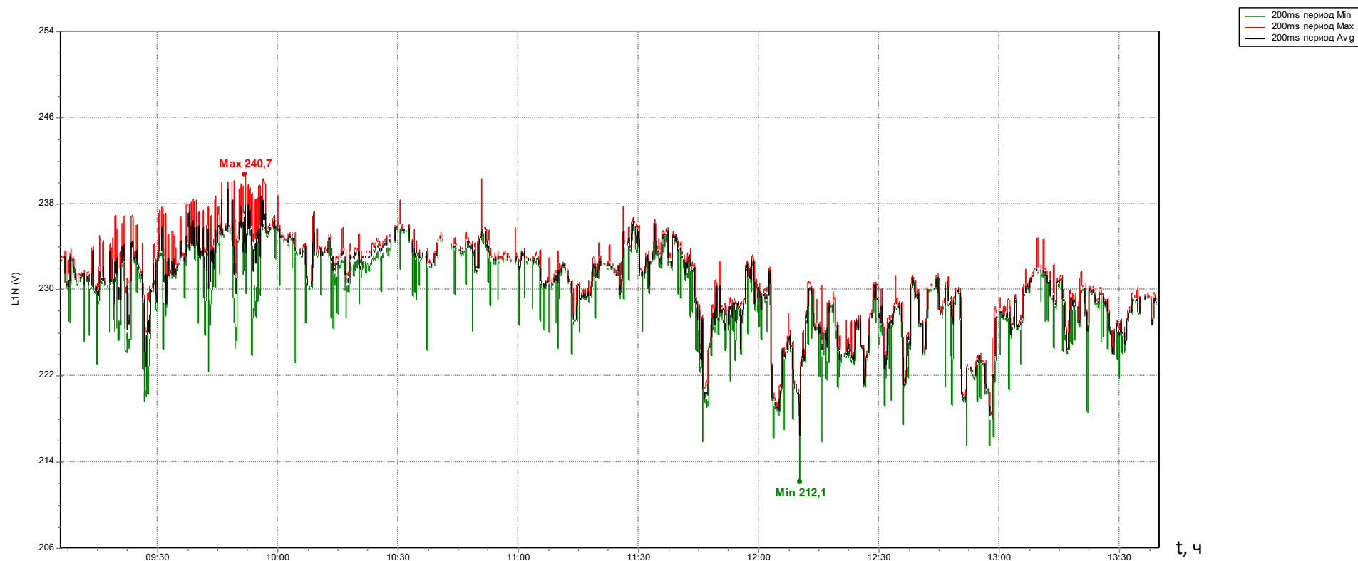
График отклонения напряжения при отключенной солнечной электростанции.
