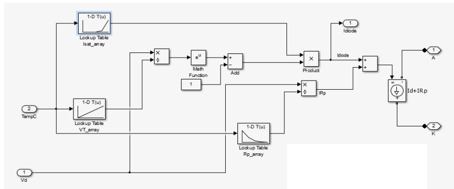
Рисунок 2.6. – Схема изменения выходных параметров шунтирующего диода.
