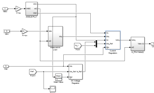
Рисунок 2.9. - Схема управления инвертором
