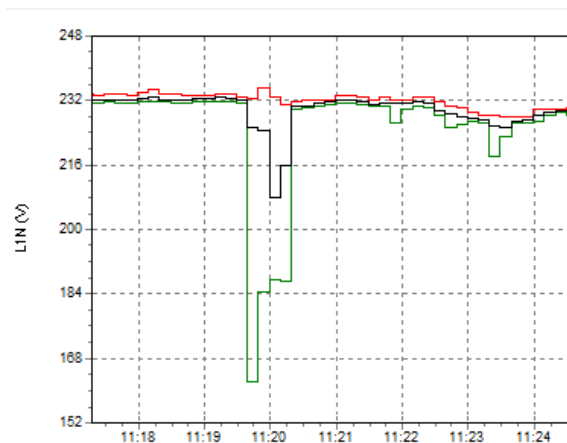
Рисунок 4.2 – Результаты эксперимента: напряжение на шинах инвертора
