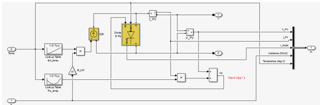
Рисунок 2.5 – Структурная схема фотоэлектрического модуля
