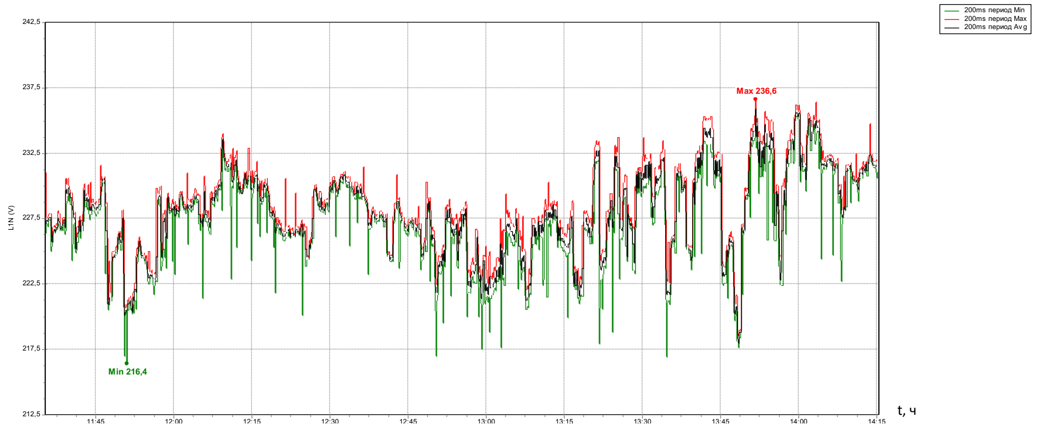
График отклонения напряжения при работающей солнечной электростанции.
