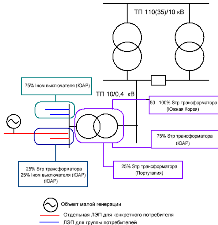
Рисунок 1.9 – Технические ограничения по подключению объектов распределенной генерации к централизованной сети.
