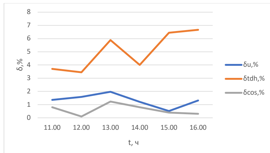
Рисунок 3.8 - Погрешность определения показателей качества электроэнергии.
