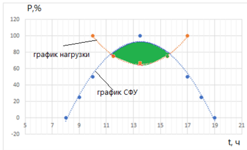
Рисунок 3.6 – График выработки СФУ и нагрузки потребителя
